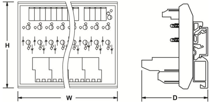
Dimensions
